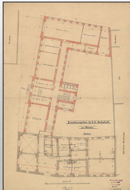
Erweiterungsbau der k.k. Fachschule zu Bozen, 1901, Stadtbauamt Obering. Peter Tecini.
