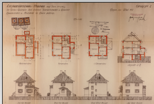
Progetto di casa unifamiliare facente parte del complesso Villenkolonie Quirain , 1912.
