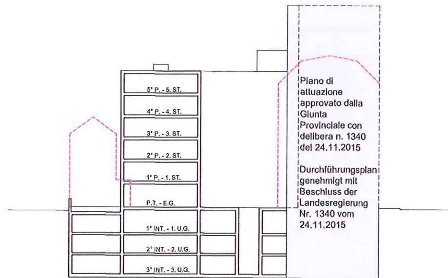
SEZIONE SCHNITT B-B
